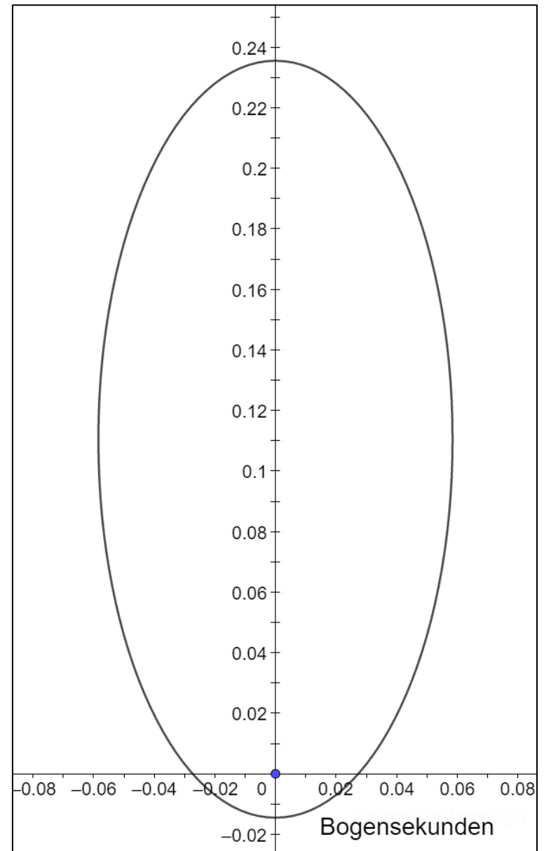
Die wahre Ellipse des Sterns S2
