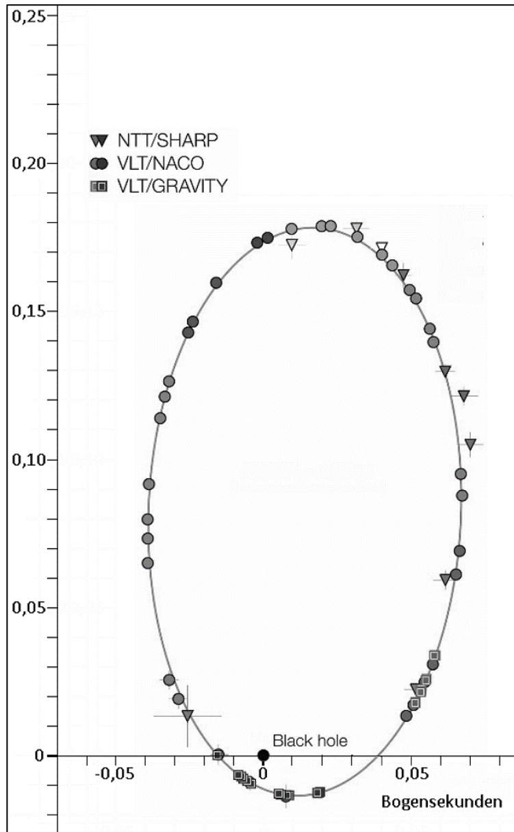
Die scheinbare Ellipse des Sterns S2
